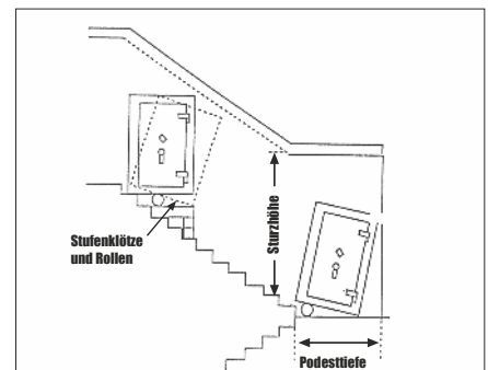
6. Treppe 180° abgewinkelt mit Podest
